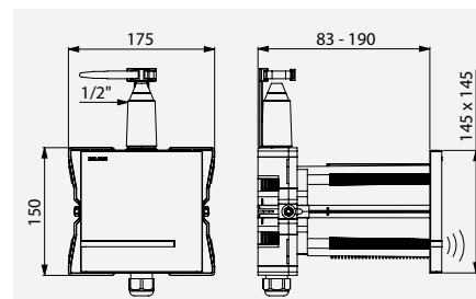
Urinalspüler TEMPOMATIC 4 für Unterputzmontage Art. DELABIE: 430PBOX + 430006
